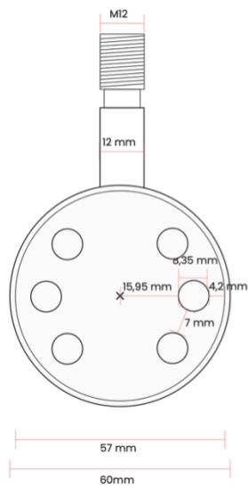
Achteraanzicht
