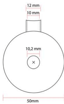
Achteraanzicht
